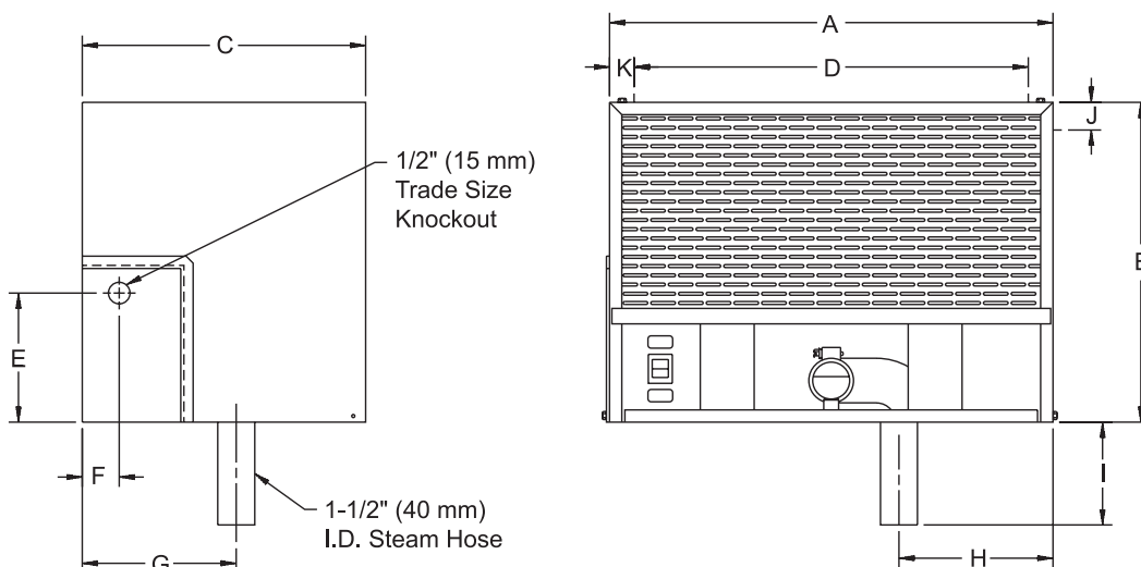
Figure 148-2. EHF-3
