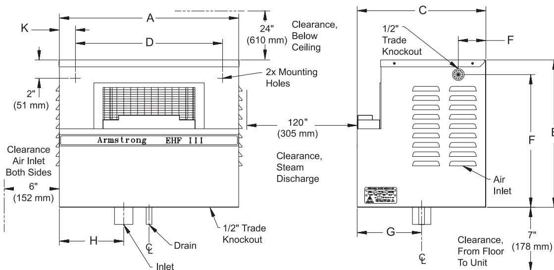
Figure 148-2. EHF-3
